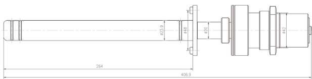
FD4426B型捻线锭子
