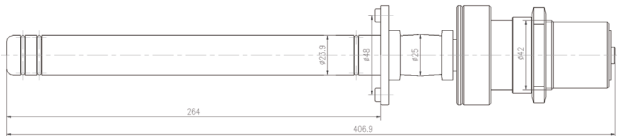
FD4425A型捻线锭子
